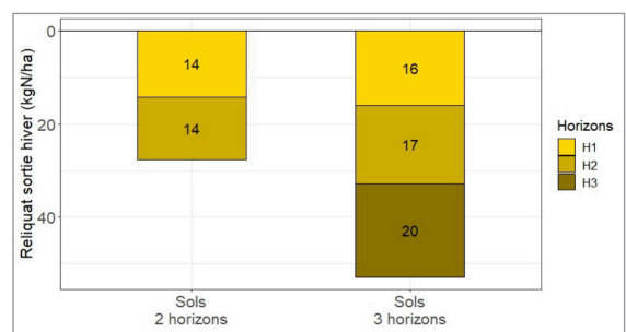
Reliquats sortie hiver 2023.
