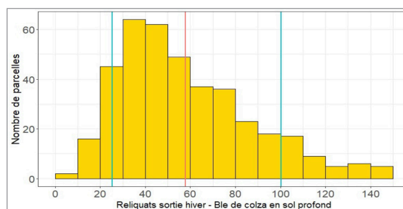
Variabilité des reliquats sortie d'hiver sous les blés de colza. Lignes bleues : 10 e et 90 e quantiles. Ligne rouge : moyenne.
